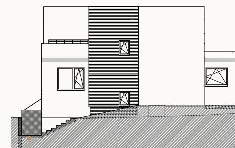
Boční pohled
